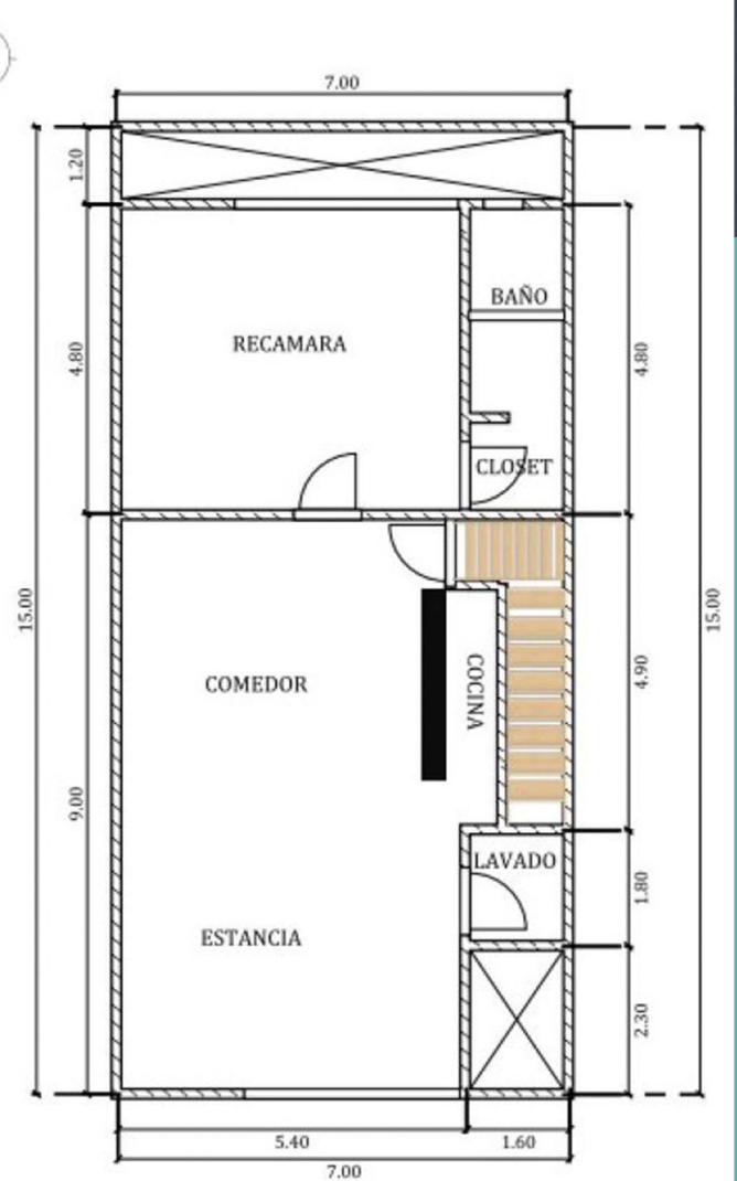
Planta alta
