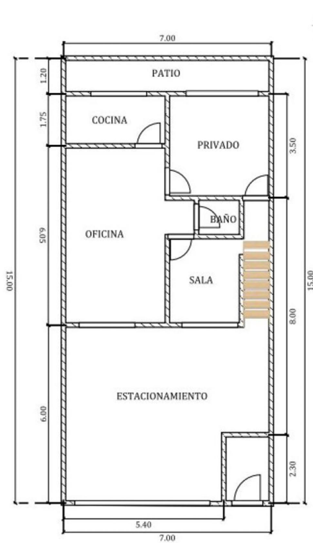
Planta baja
