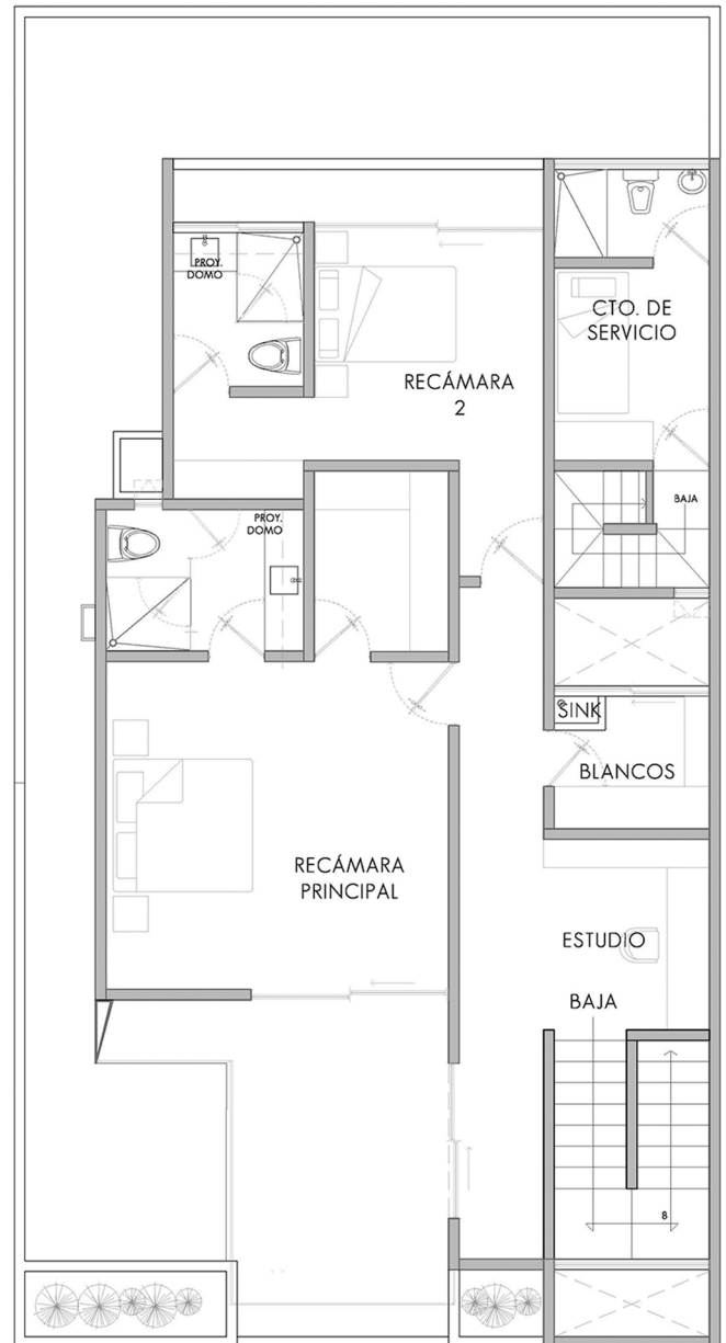
PLANTA ALTA
